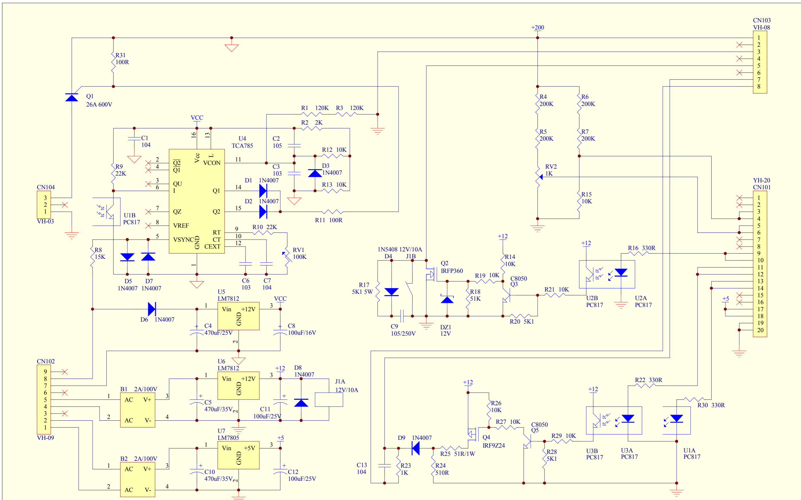
SW2500控制电路原理图
